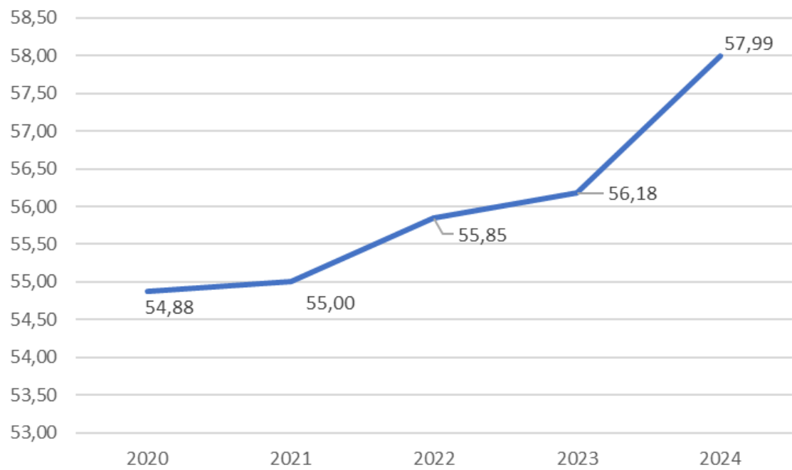
Grafik II.47 Persentase Jaringan Irigasi Dalam Kondisi Baik Kabupaten Trenggalek Tahun 2020-2024
